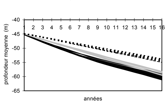
Figure 8. Comparaison de la profondeur de nappe entre le scénario actuel et 2 scénarios d'intervention par le prix.
