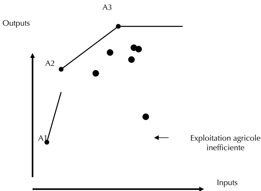
Figure 2. Enveloppe linéaire par morceau.
