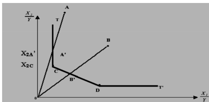
Figure 3. La forme ratio du modèle CCR.
