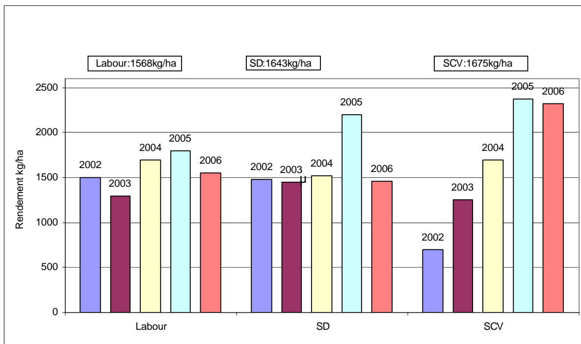
Figure 1. Comparaison des rendements de coton entre 3 systèmes de culture à Windé de 2002 à 2006 : fumure vulgarisée.
